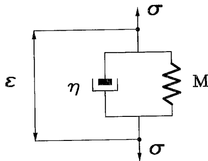
Kelvin-Voigt Model
